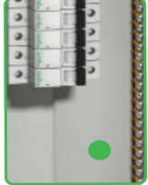
أقطاب تأريض أقطاب حيادية Terminal Block for Earth and neutral
