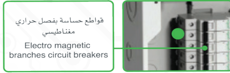
من ١٢ - ٤٢ خط From 12 to 42 way
